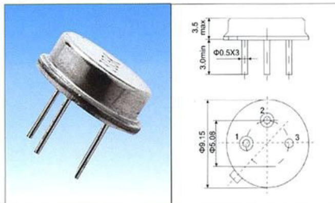
TO39
